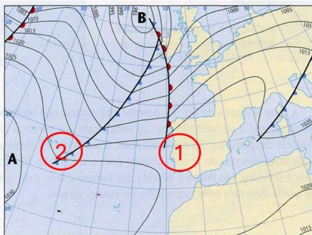
Figura 1 – Esquema sinóptico para uma situação típica de inverno
